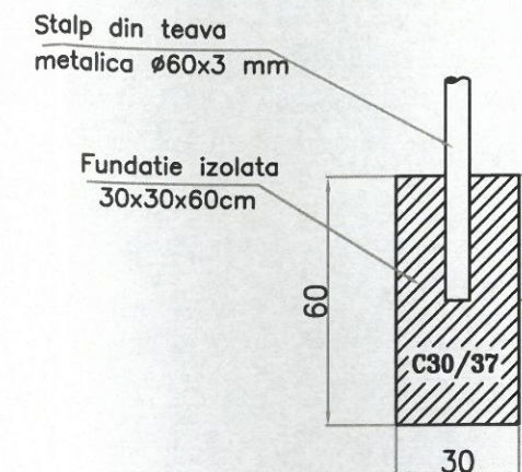
SECTIUNE A-A Scara 1:10
