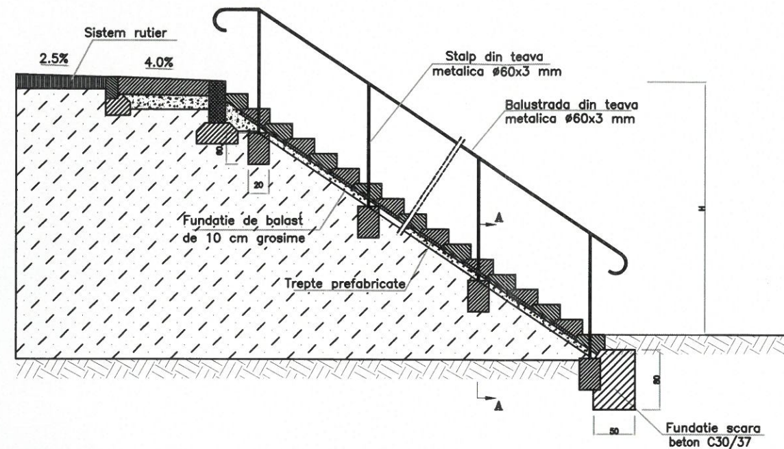
SECTIUNE TRANSVERSALA Scara 1:50
