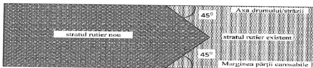
b) Racordarea în plan
