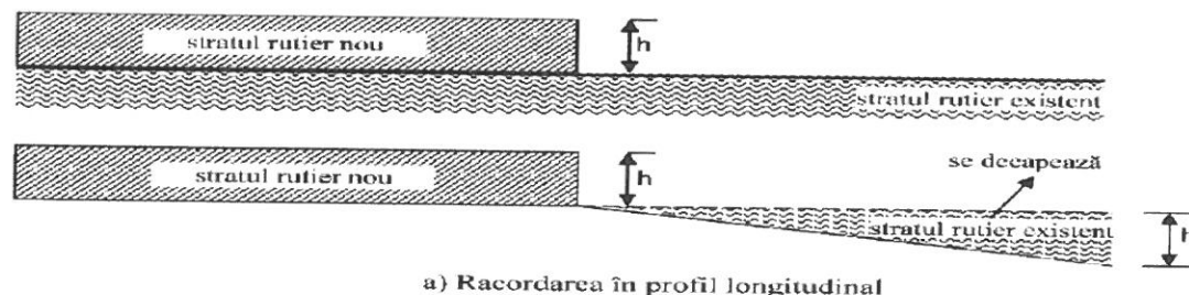
Fig. 1 Racordarea stratului rutier nou cu stratul rutier existent
