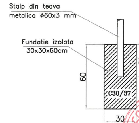
SECTIUNE A-A Scara 1:10
