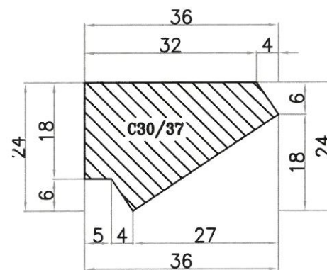
SECTIUNE TRANSVERSALA
