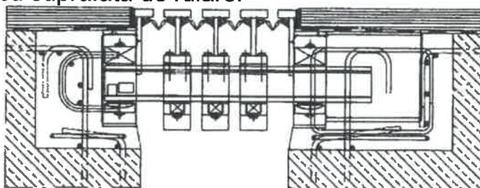
Fig. 8 Sectiune transversala rost de dilatatie modular cu traversa cu elemente de control de forfecare cu arcuri. (TIP C)
