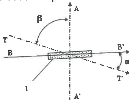
Fig. 16: Definierea direcției de deplasare și abaterilor de la aceasta, pentru determinarea deplasării descendente/coborare
