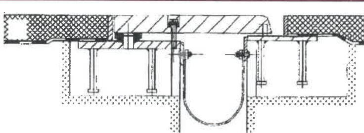
Fig.6 Sectiune transversala prin rost de dilatatie tip Finger (pieptene glisant)
