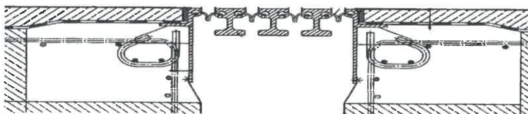
Fig.9 Sectiune transversala rost de dilatatie modular cu traversa cu elemente de control de forfecare cu arcuri intre grinzile centrale, pentru suprafata carosabila.
